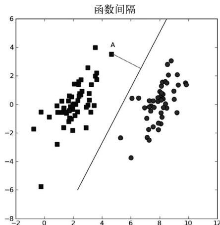
图6-3 点A到分隔平面的距离就是该点到分隔面的法线长度
