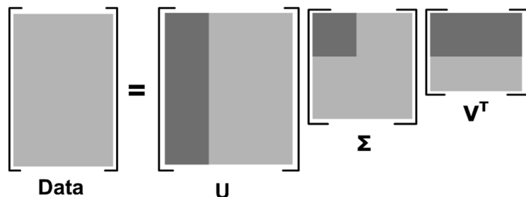
图14-2 SVD的示意图。矩阵Data被分解。浅灰色区域是原始数据，深灰色区域是矩阵近似计算仅需要的数据
