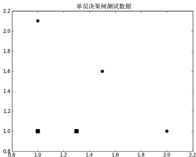
图7-2 用于检测AdaBoost构建函数的简单数据。这不可能仅仅通过在某个坐标轴上选择某个阈值来将圆形点和方形点分开。AdaBoost需要将多个单层决策树组合起来才能对该数据集进行正确分类
